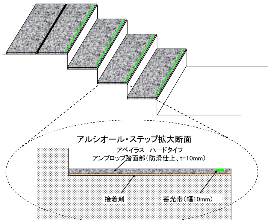
図. 1 階段部全体施工断面図
