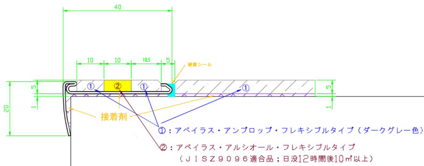
図. 2.2 アルシオール ステップ テーパー無し断面図
