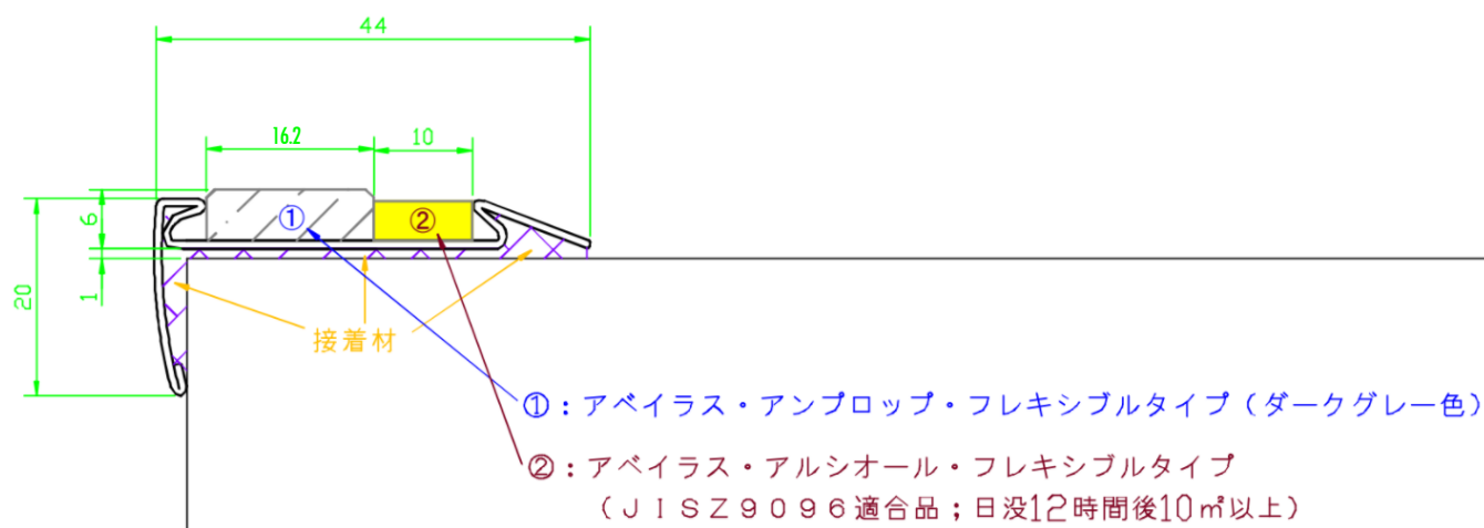
図. 2.1 アルシオール ステップ テーパー有り断面図
